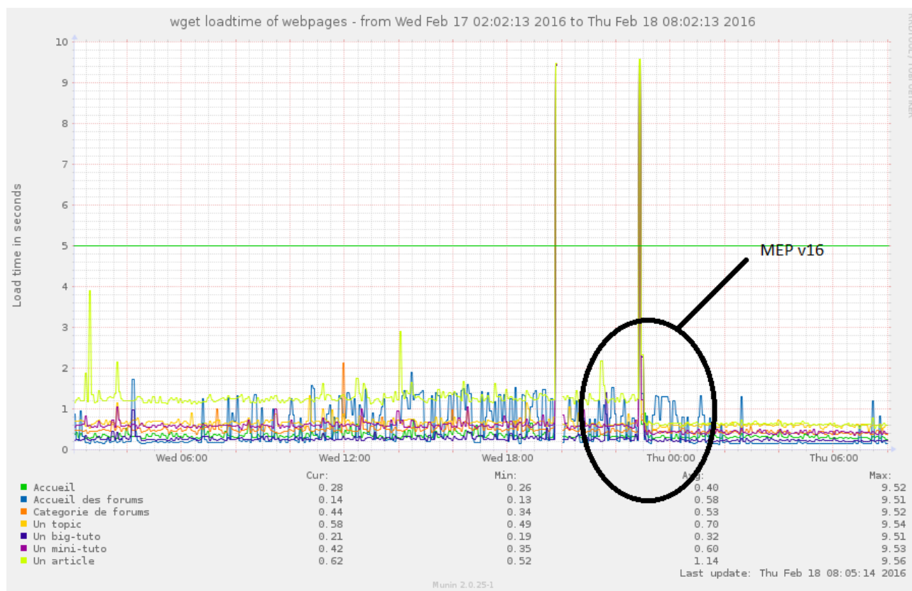
FIGURE 2. – Amélioration significative des performances sur la v16
