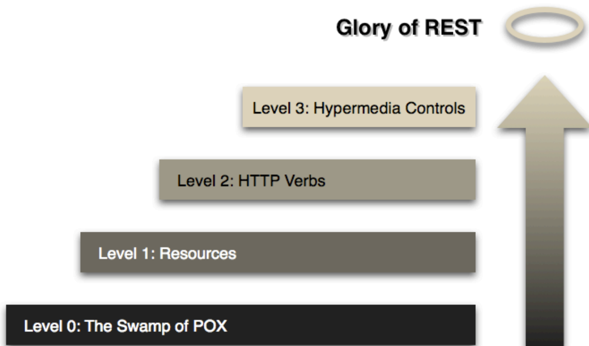
Figure 4.1 – Le modèle de maturité de Richardson mis en image par Martin Fowler
