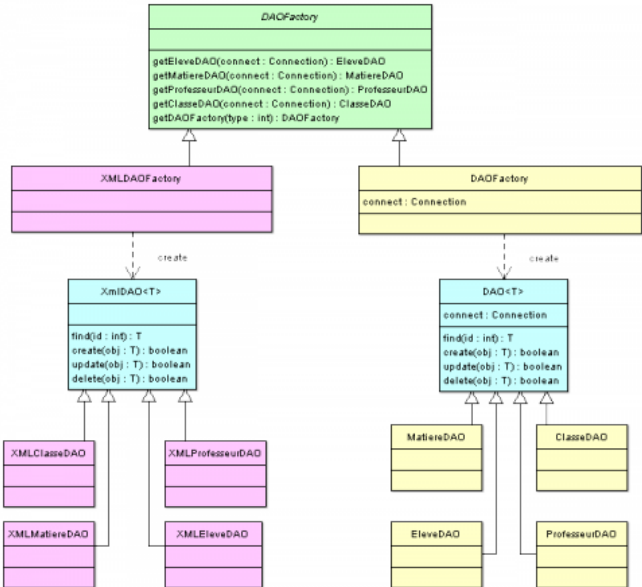
FIGURE IV.5.10. – Diagramme de classe de nos factory
