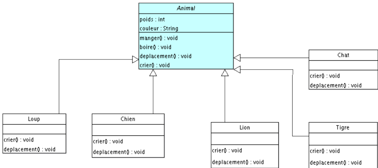
FIGURE II.5.2. – Hiérarchie de nos classes
