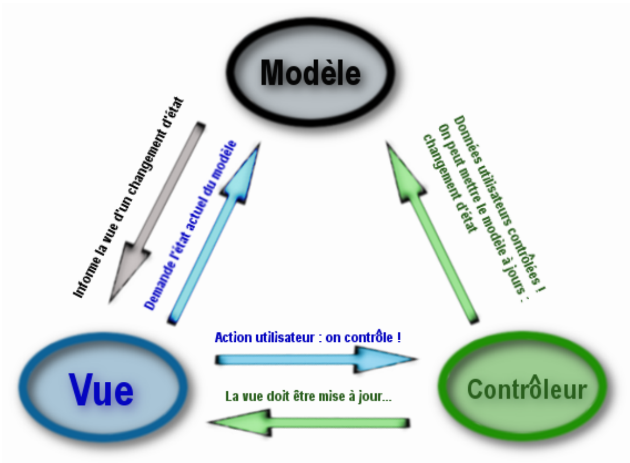
FIGURE III.14.1. – Schéma du pattern MVC
