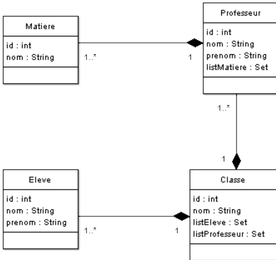
FIGURE IV.5.1. – Diagramme de classe de notre BDD
