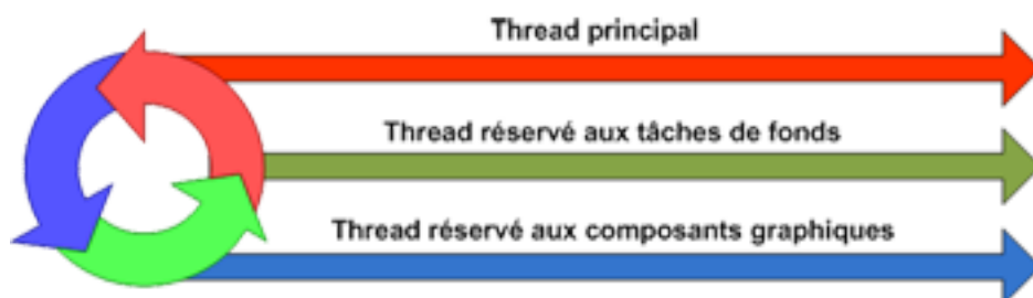
FIGURE III.16.1. – Threads lancés au démarrage de tout programme Java
