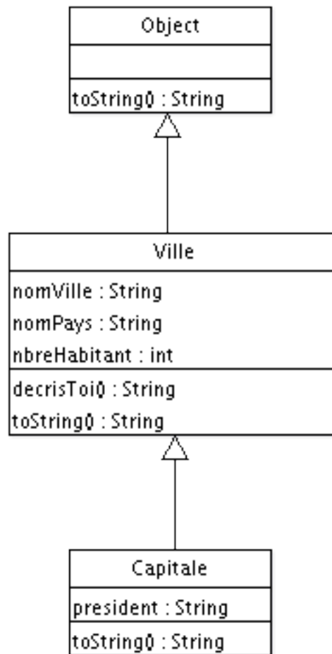
FIGURE II.3.1. – Exemple de diagramme de classes
