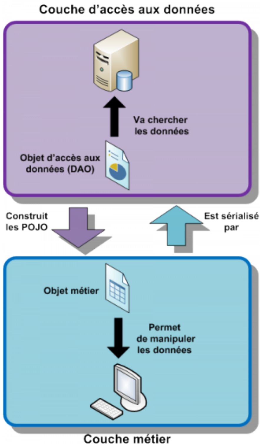
FIGURE IV.5.2. – Fonctionnement du pattern DAO
